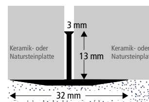
Fugenprofil
